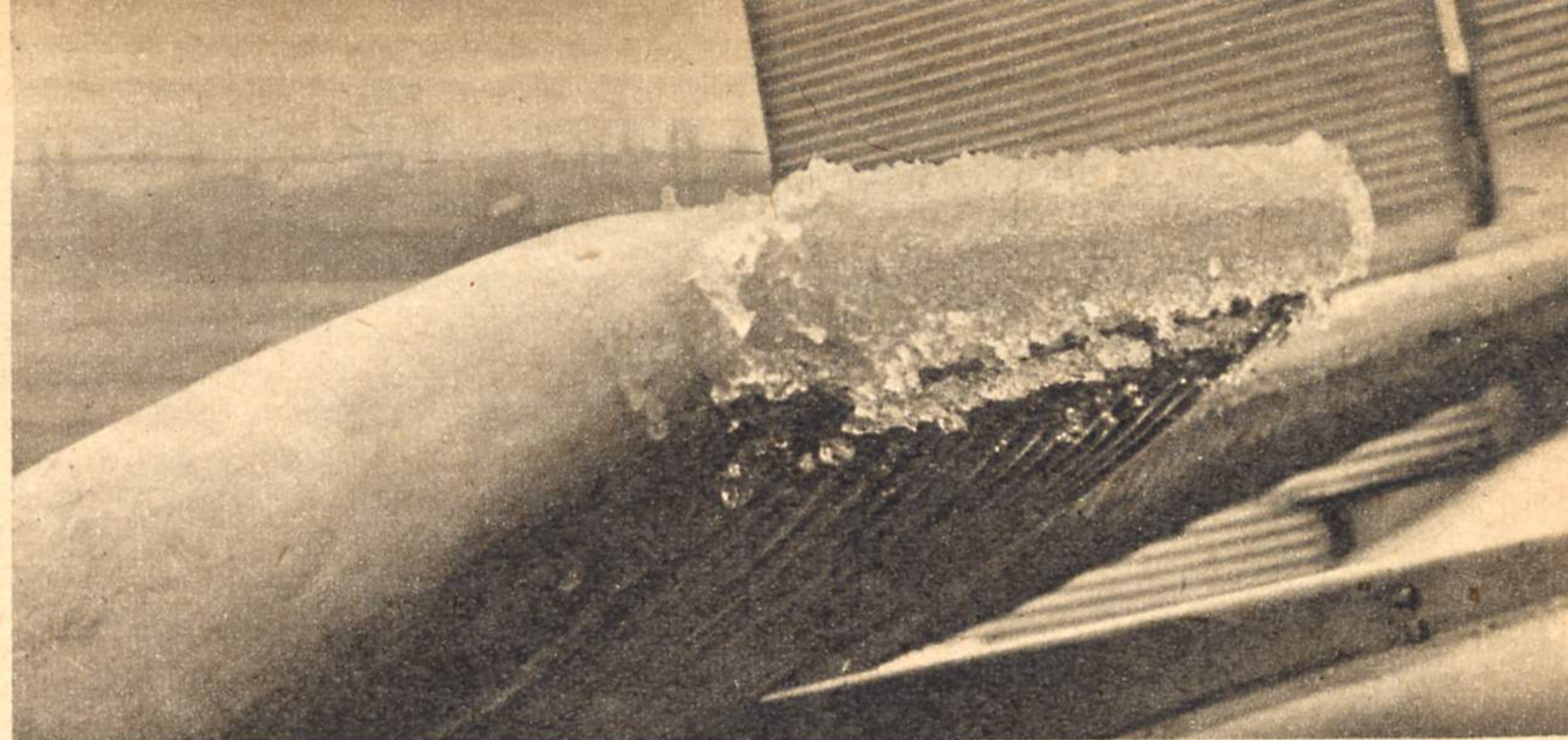
Vereiste Vorderkante des Höhenruderausgleichs einer Ju 52
