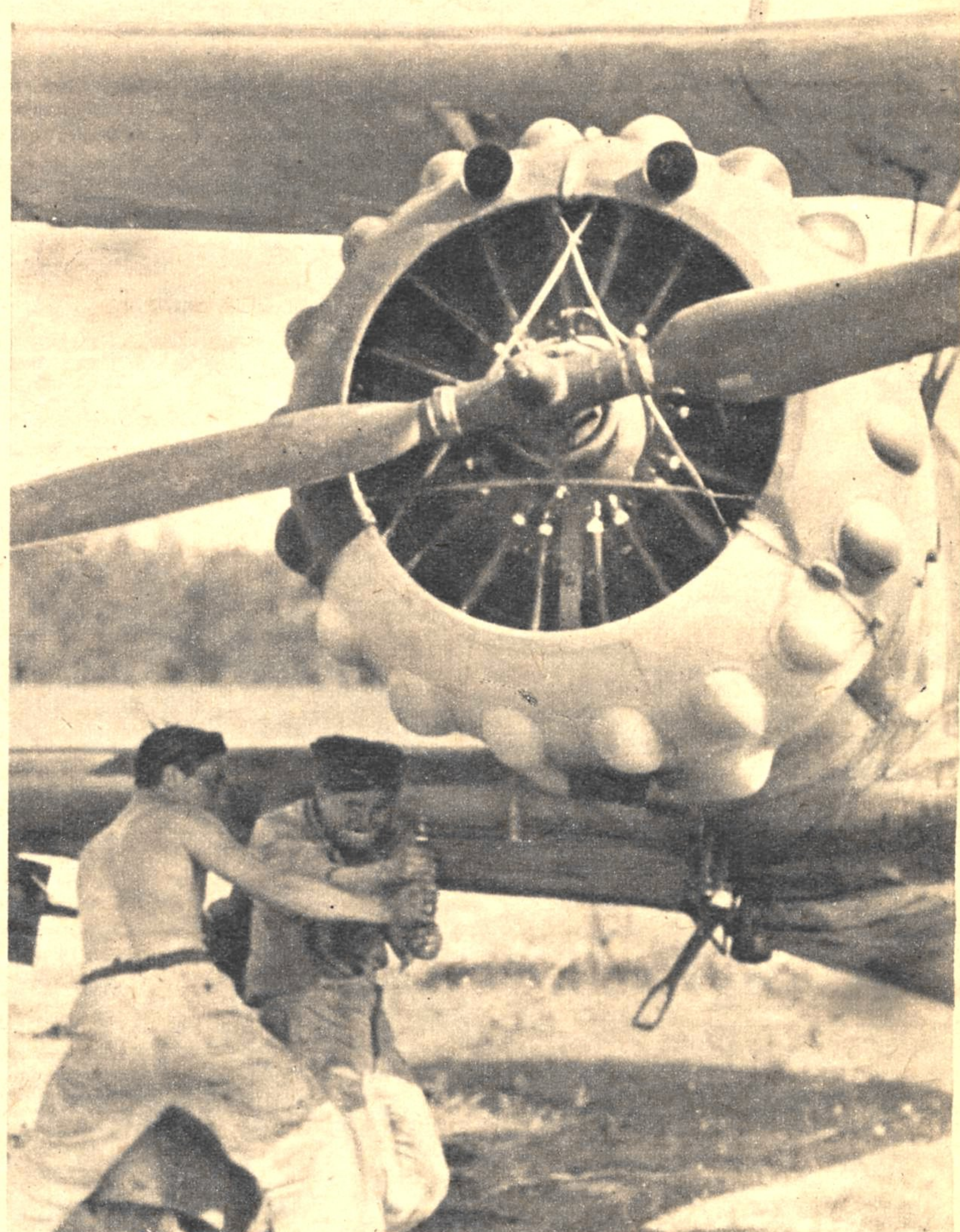
Das Gesicht des Schlachtflyers. Die gewaltige Motorhaube gibt dem Sturzkampfeinsitzer Hs 123 mit seinem festen und gedrunghen Rumpf das charakteristische Gepräge. Männer vom Bodenpersonal beim Anwerfen des Motors kurz vor dem Start
